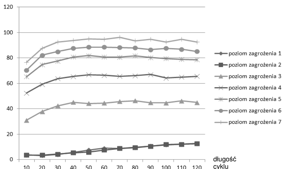
Rys. 4. Liczba zatrzymań dla zdefiniowanych poziomów zagrożeń Fig. 4. Average stops number for a defined weather threat level
