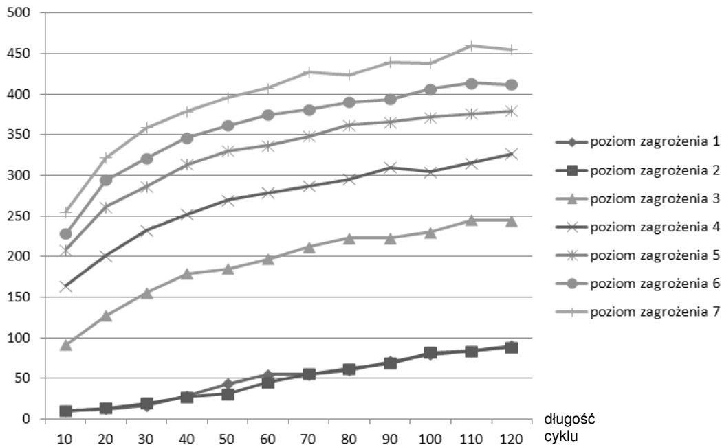
Rys. 3. Średnie straty czasu zatrzymania dla zdefiniowanych poziomów zagrożeń Fig. 3. Average stop delays for defined weather threat level
