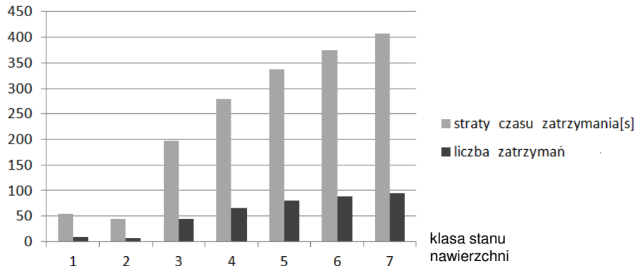
Rys. 2. Średnie straty czasu zatrzymania oraz średnie liczby zatrzymań dla cyklu równego 60 s Fig. 2. Average number of stops and average delays for a cycle equals 60 s
