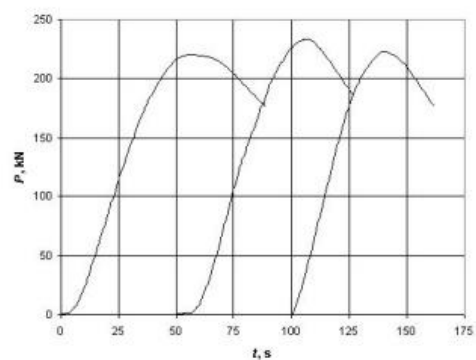
Rys. 15. Zależność siły w funkcji czasu dla WZ2 Fig. 15. Force dependence in time function for WZ2
