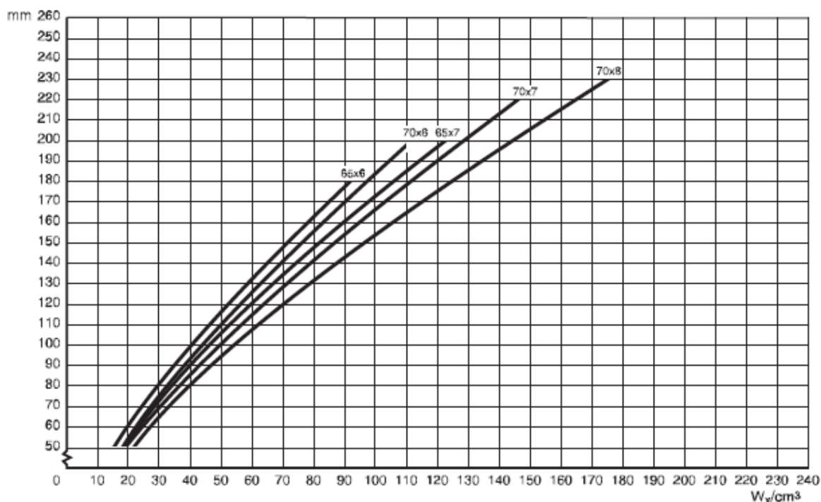
Rys. 3. Funkcje wymiarów profili na podłużnice ramy montażowej w konstrukcji profilu otwartego [4] Fig. 3. Functions of the profiles for the side dimensions of the mounting frame in the construction of an open structure [4]
