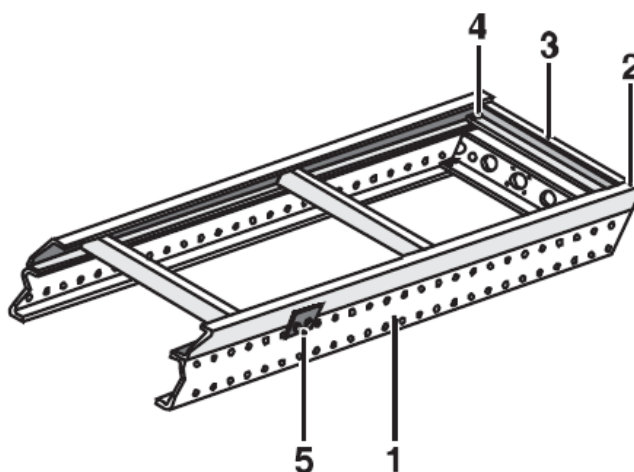
Rys. 5. Mocowanie ramy montażowej: 1 – rama podwozia, 2 – rama montażowa, 3 – poprzecznicą, 4 – śruby do unieruchomienia wzdłużnego, 5 – płyta prowadząca, do unieruchomienia poprzecznego [4]
