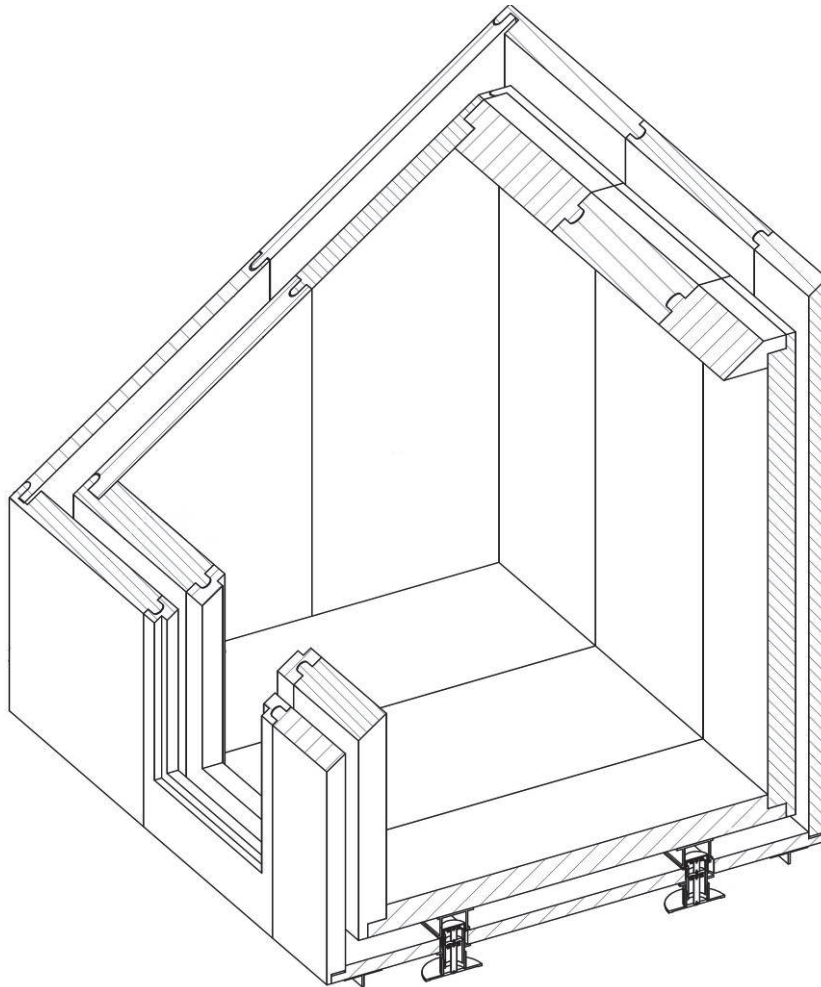
Rys. 1. Schemat kabiny izolowanej akustycznie Fig. 1. The scheme of the cabin with acoustic insulation
