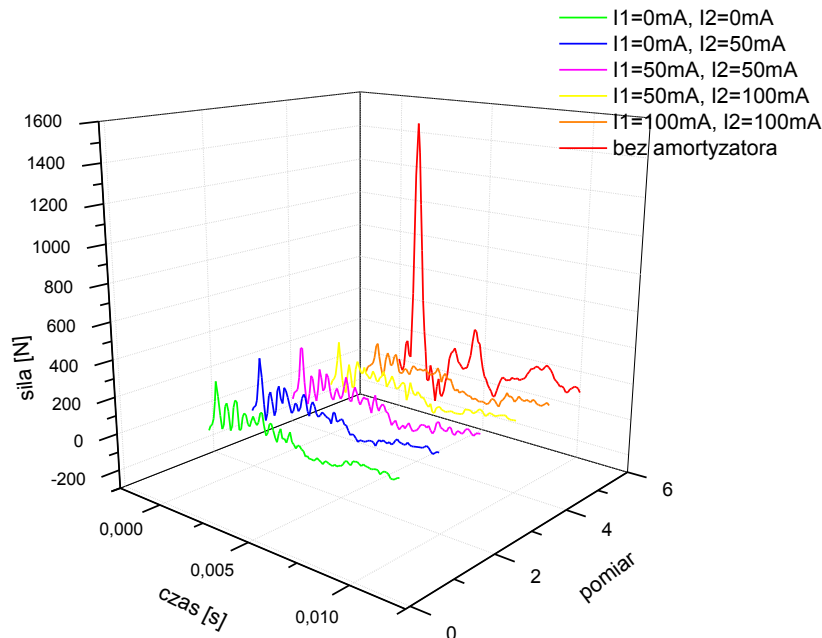
Rys. 5. Porównanie sił występujących w układzie karabin–strzelec bez tłumików MR i z tłumikami przy prądach sterowania tłumika suwadła I_1 = 0 mA i tłumika kolby I_2 = 50 mA; nabój bojowy Fig. 5. Forces acting in the rifle-shooter system for single shot mode, without dampers and with dampers for current I_1 = 0 mA for slide damper and I_2 = 50 mA for stock damper; combat bullet
