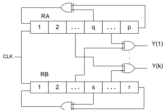
Rys. 3. Schemat generatora na dwóch rejestrach przesuwających
