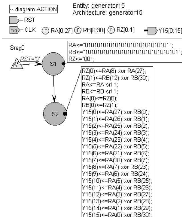
Rys. 4. Specyfikacja generatora w edytorze grafów przejść FSM
