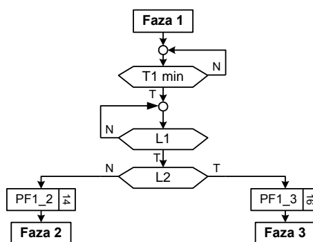
Rys. 3. Fragment algorytmu sterowania ruchem na skrzyżowaniu
