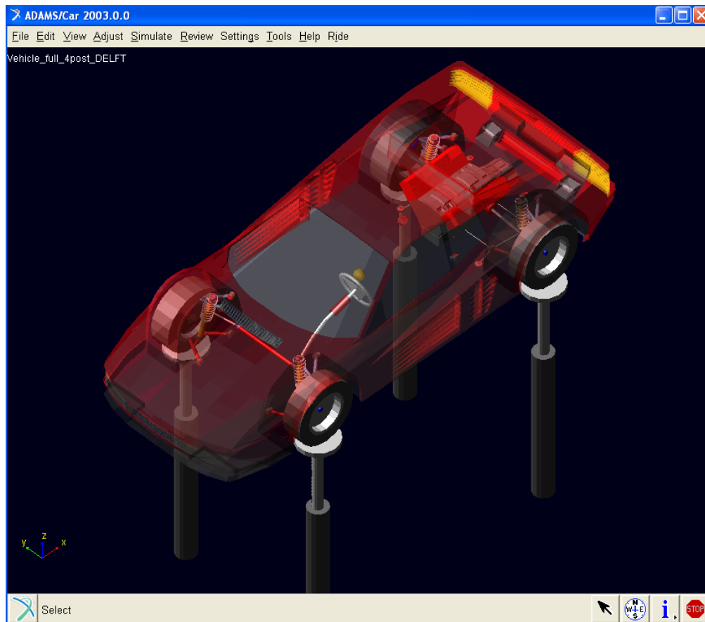
Rys. 1. Widok pojazdu na stanowisku płytowym Fig. 1. View of full vehicle on four post test rig
