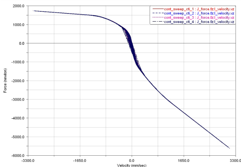
Rys. 5. Wykresy: a) wymuszenie – przemieszczenie z liniowo narastającą częstotliwością, b) wykres sił w funkcji przemieszczenia, c) wykres sił w funkcji prędkości
