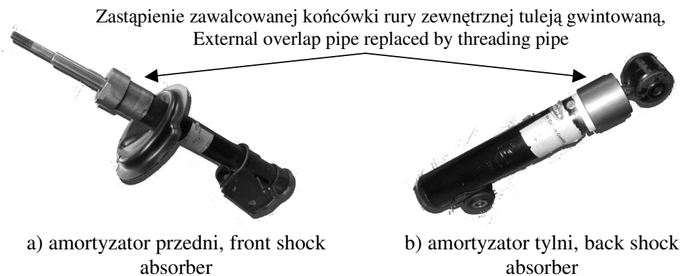
Rys. 3. Przerobiona konstrukcja amortyzatora
